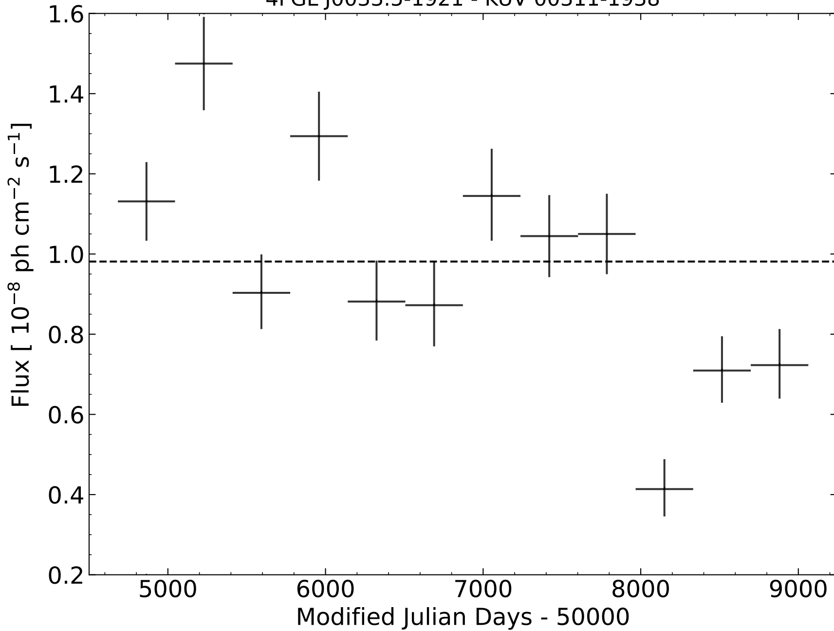
4FGL J0033.5-1921 - KUV 00311-1938
